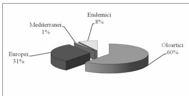
Fig. 6 - Distribuzione percentuale dei corotipi.
